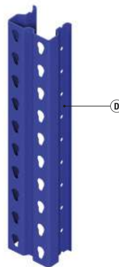
Cross Aisle Post TD U314 (Family code PU314TD)
